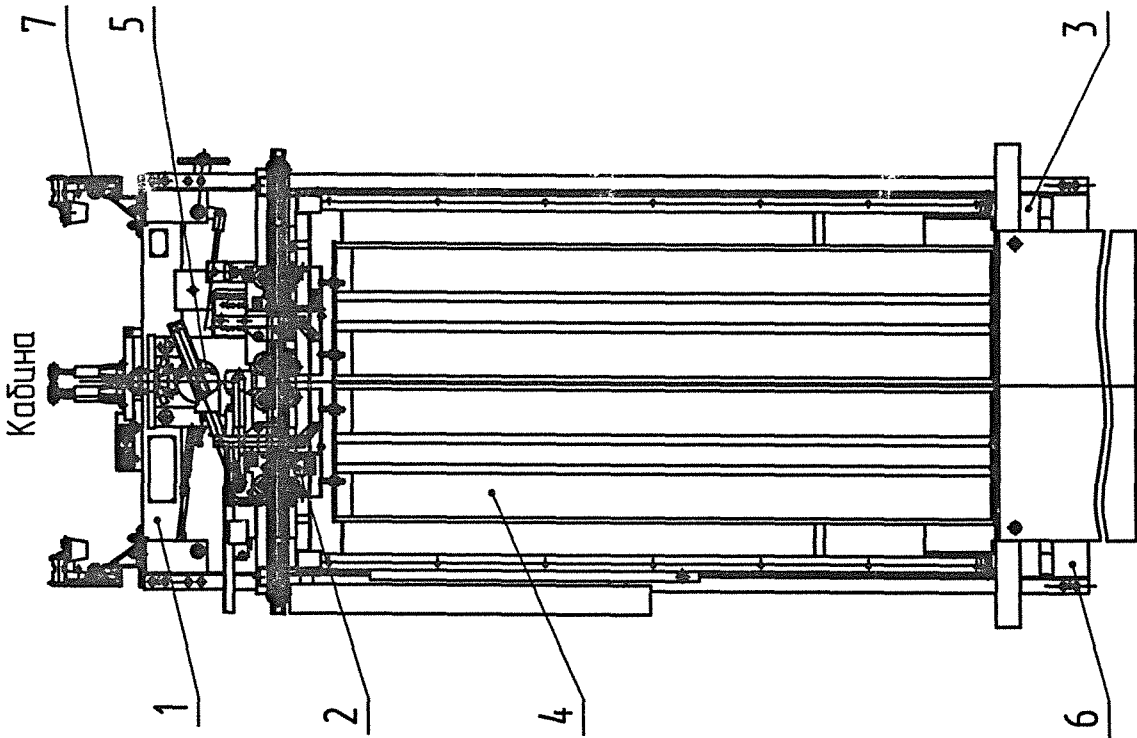
1- балка верхняя; 2- потолок; 3- пол; 4- створки дверей кабины; 5- привод дверей кабины; 6- балка нижняя; 7- башмак скользящий
