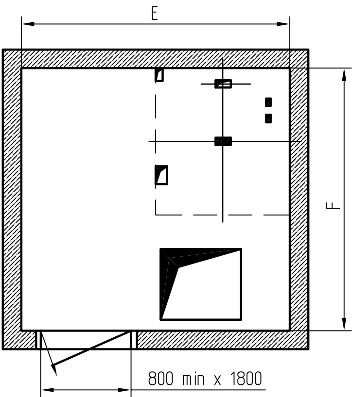
План машинного помещения
