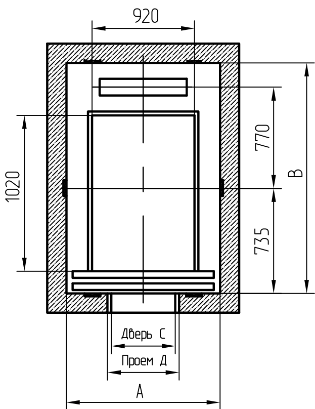
План шахты - вариант 1
