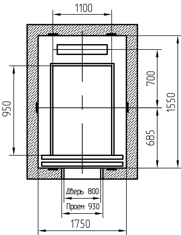
План шахты - вариант 2
