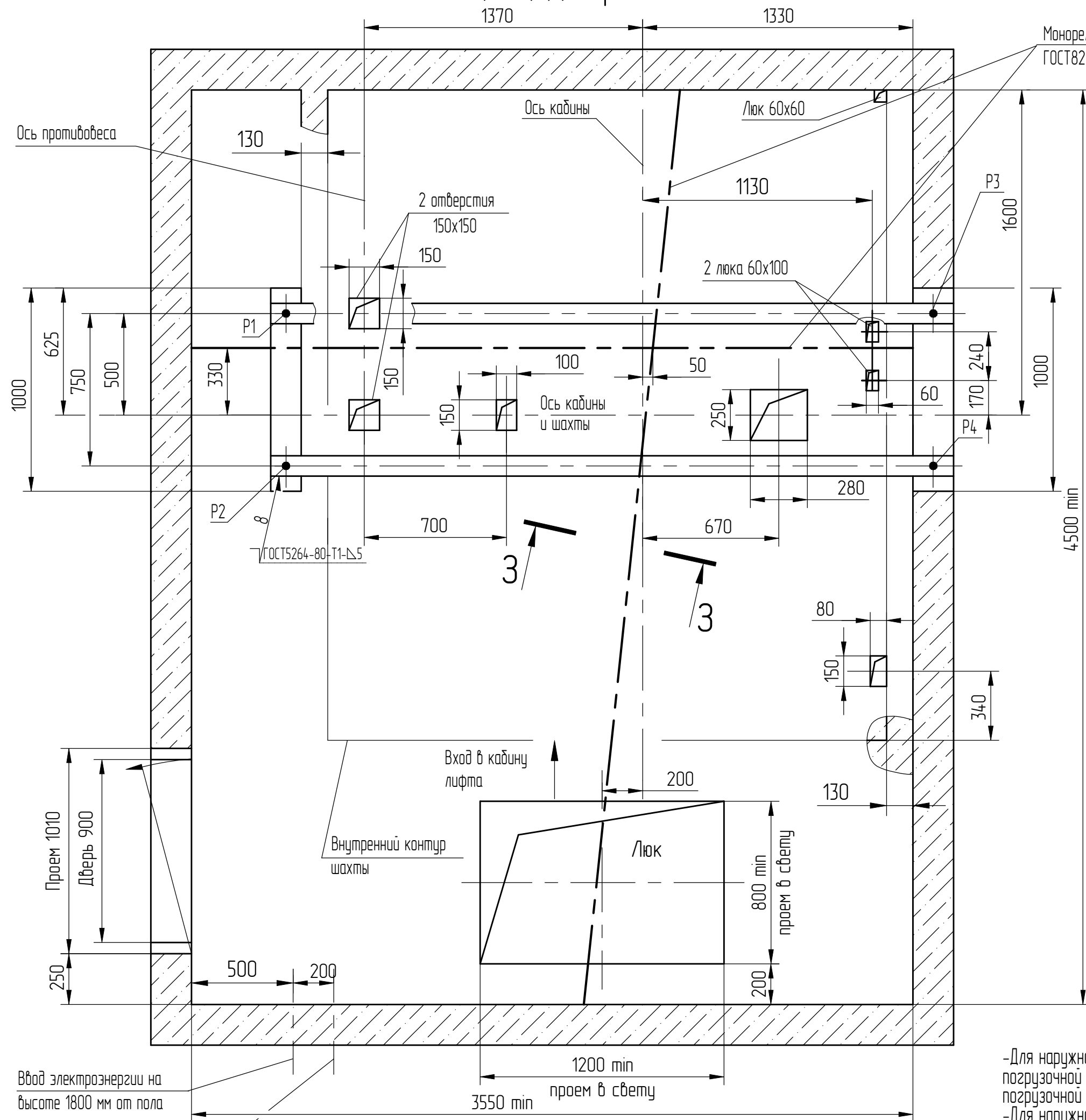
В-В (1:20) (1) Вариант 1
