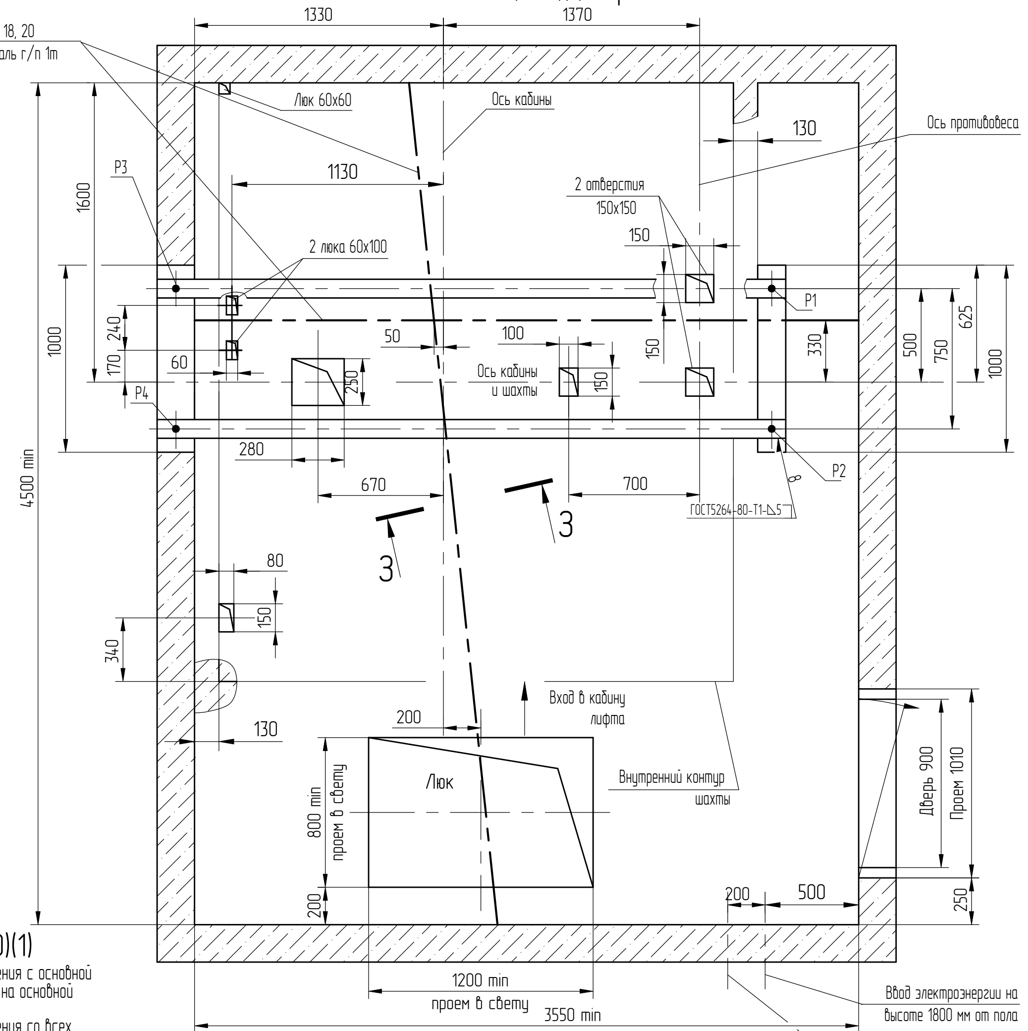
В-В (1:20)(1) Вариант 2
