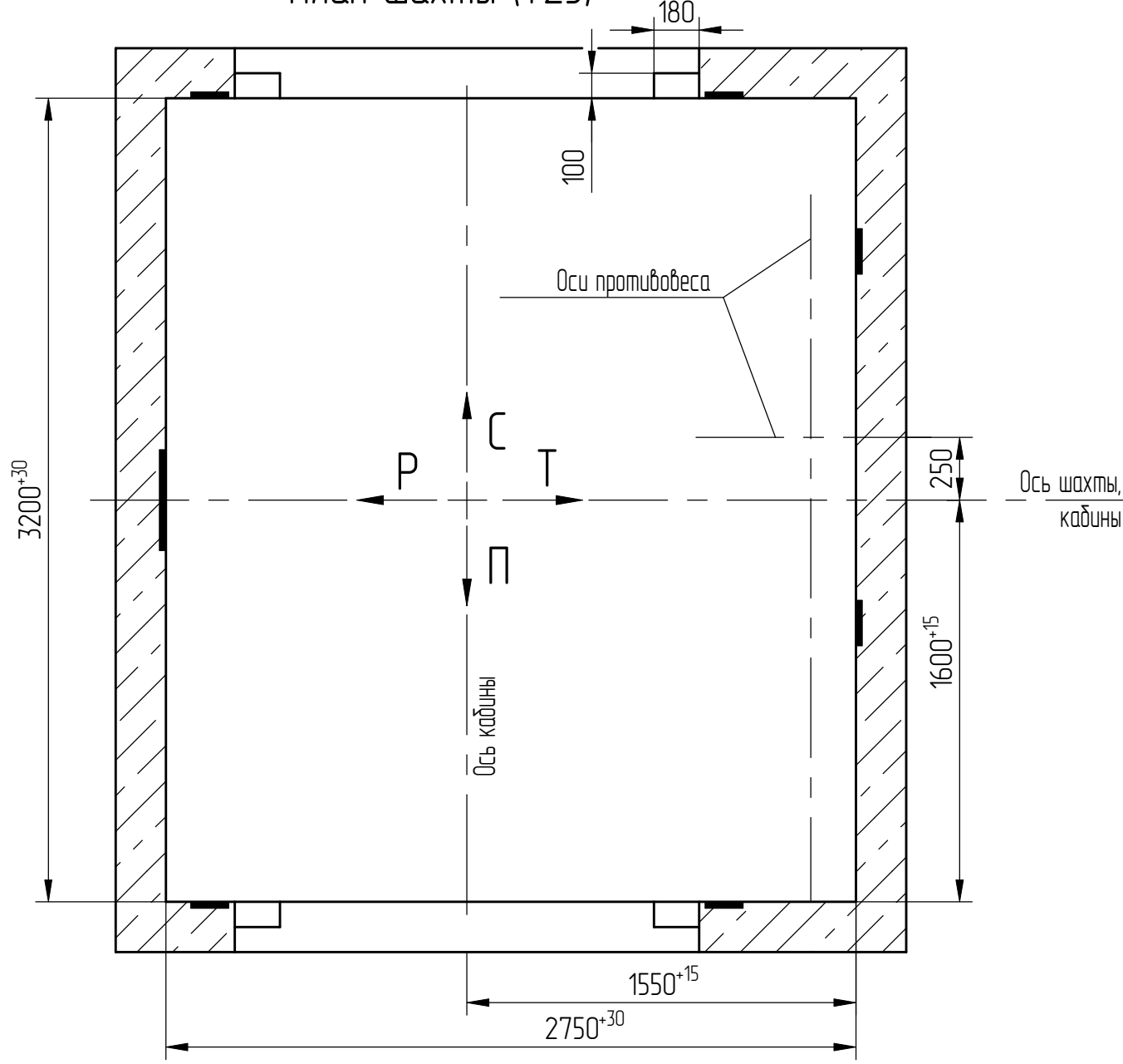
План шахты (1:25)
