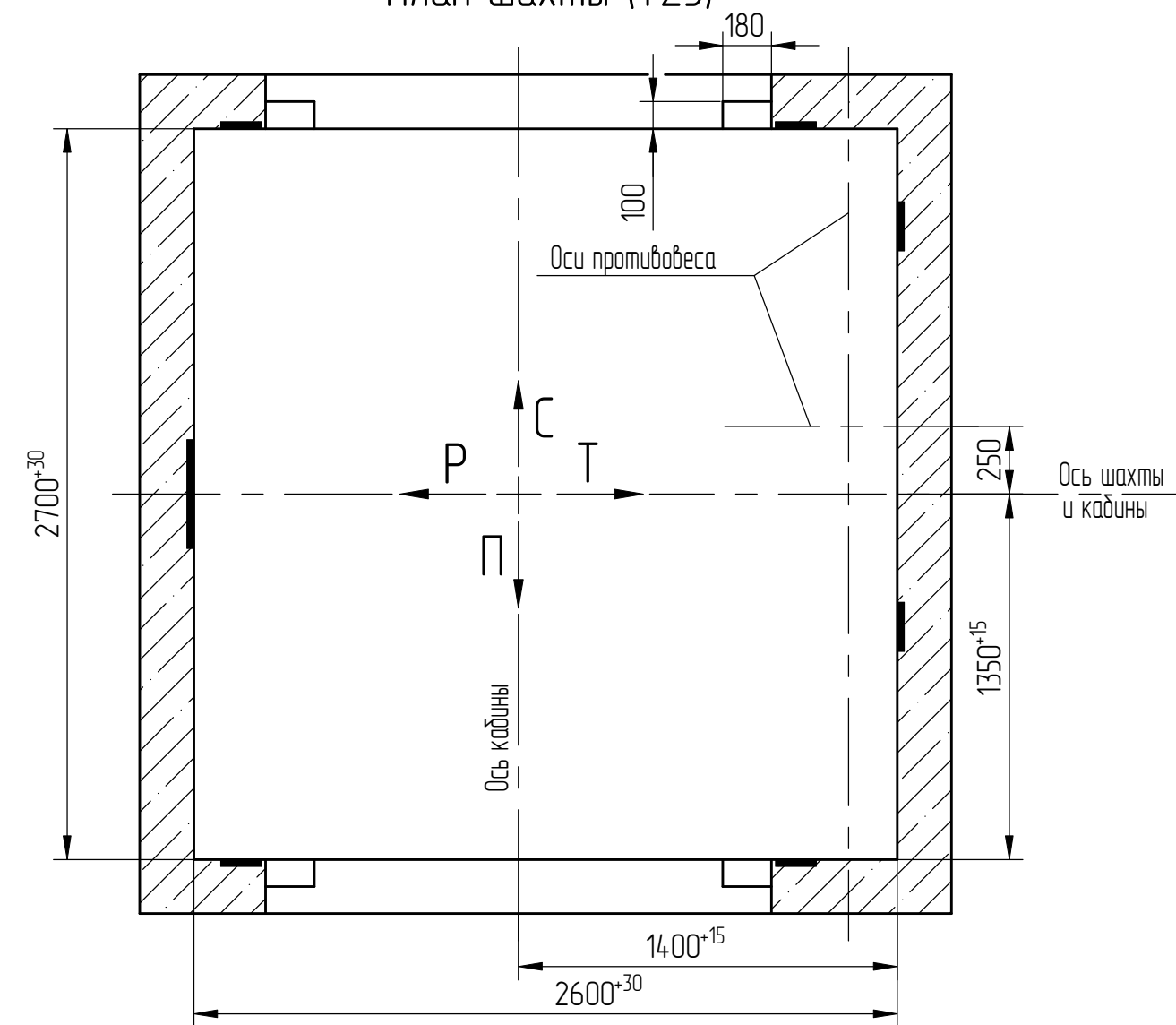
План шахты (1:25)
