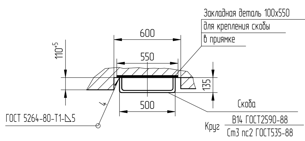
Ю-Ю (1:20)
