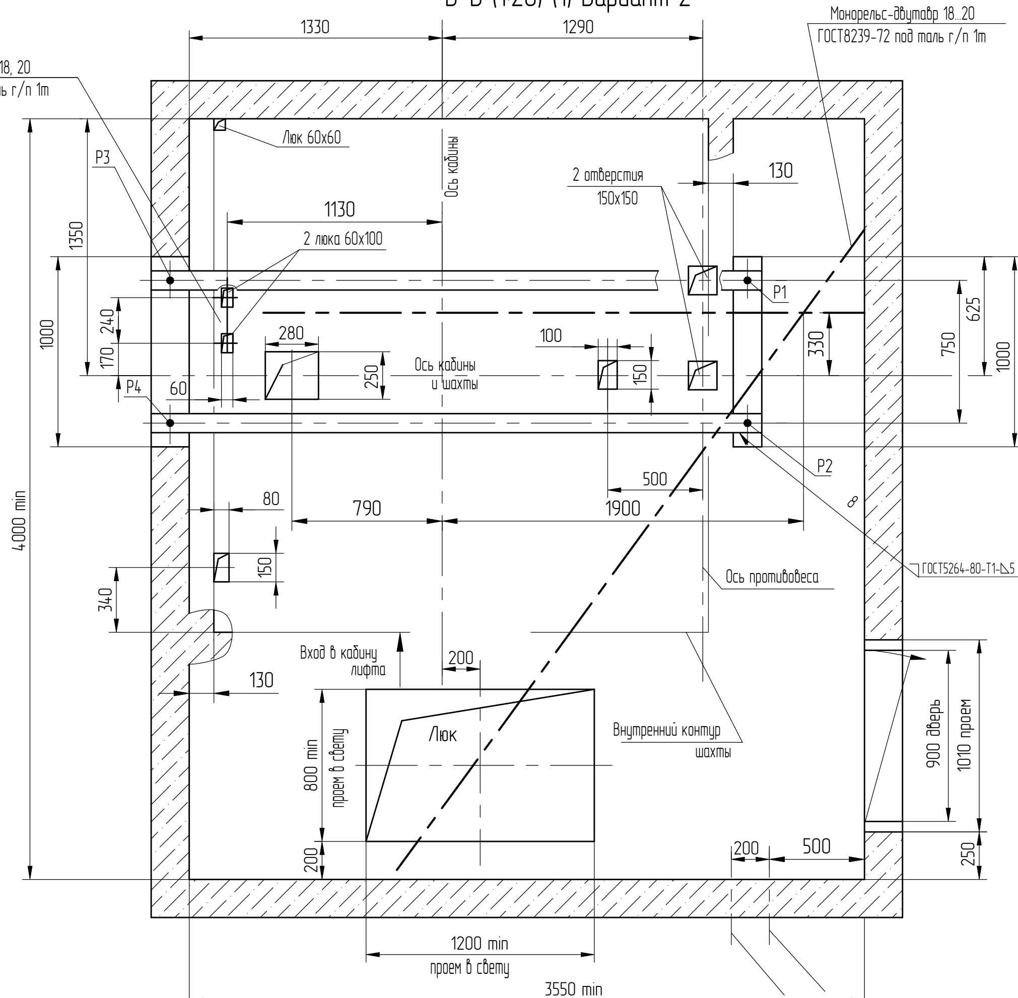
В-В (1:20) (1) Вариант 2
