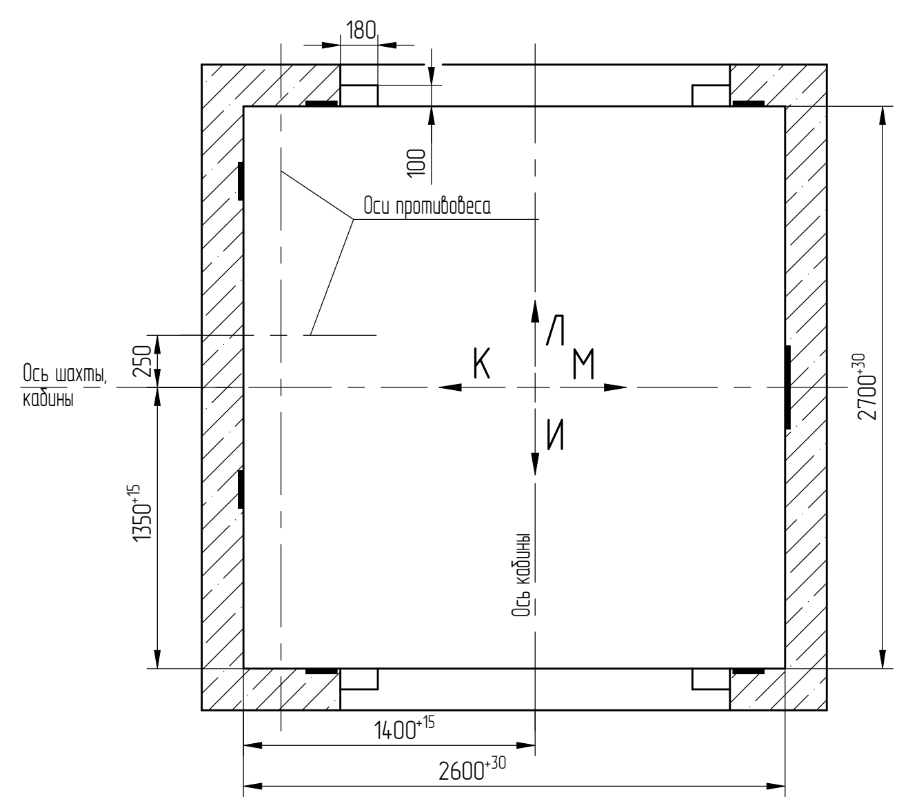
План шахты
