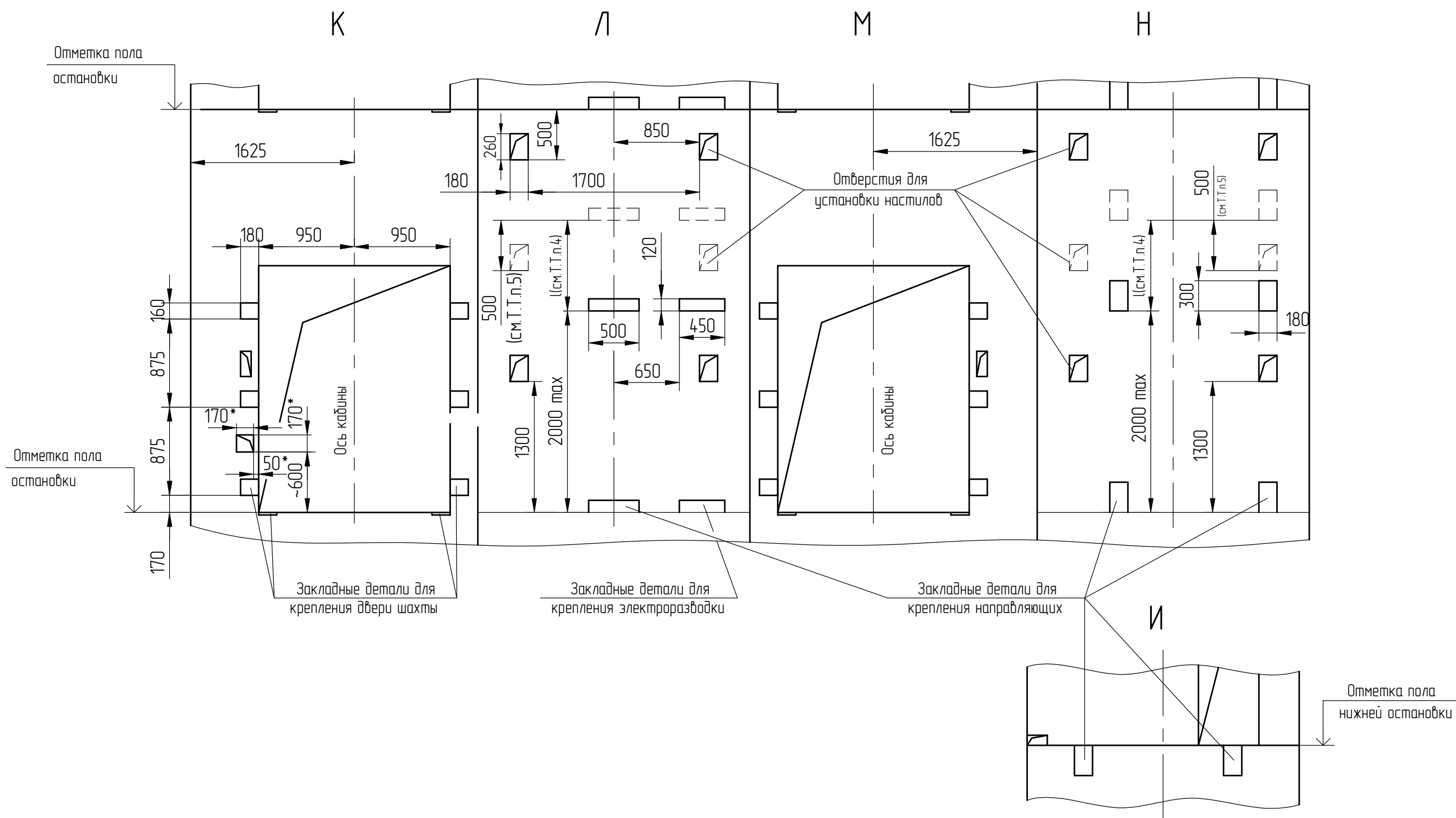
Развертка типового этажа шахты с закладными деталями. Вариант 2 (1:40)
