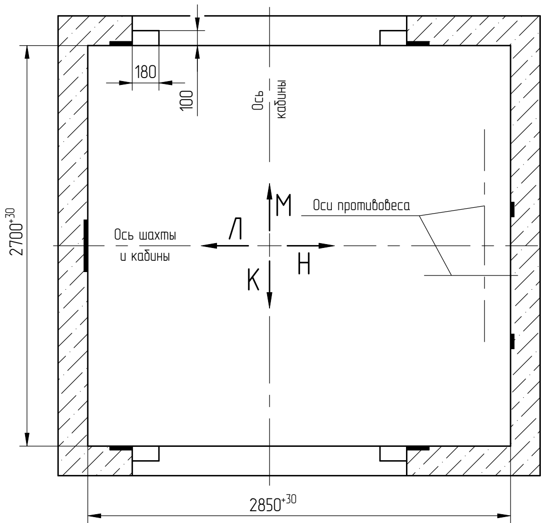
План шахты (1:25)
