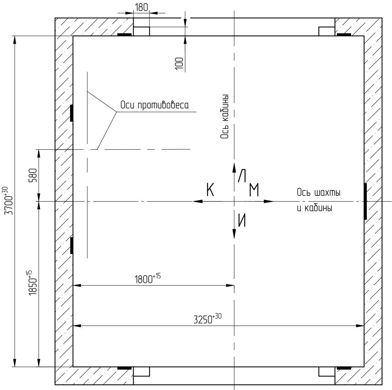
План шахты (1:25)
