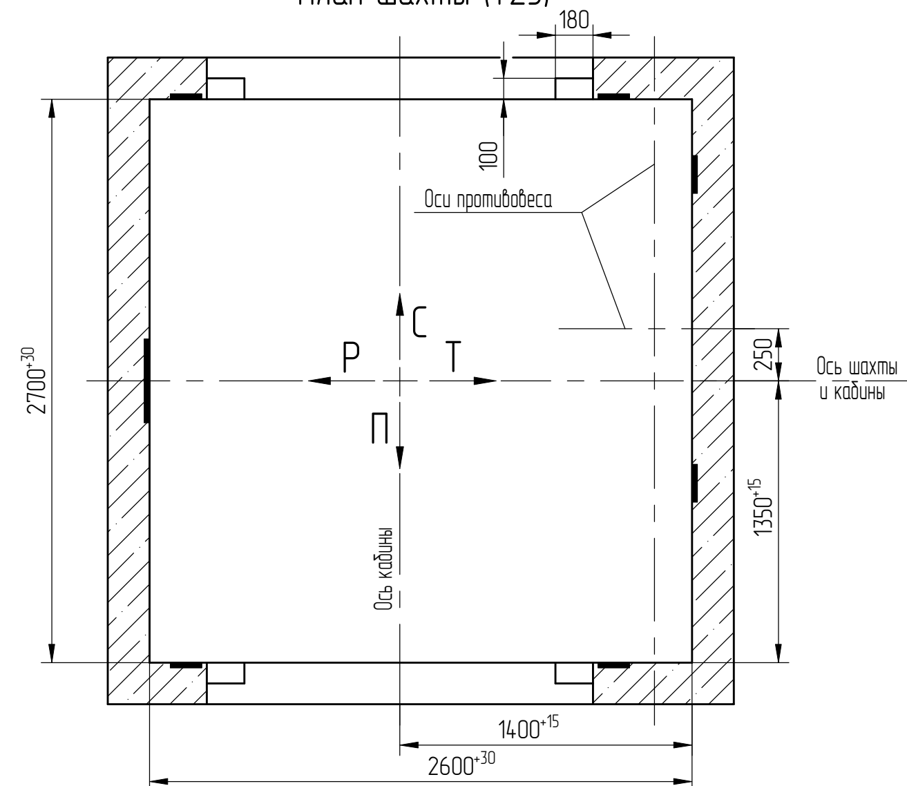
План шахты (1:25)
