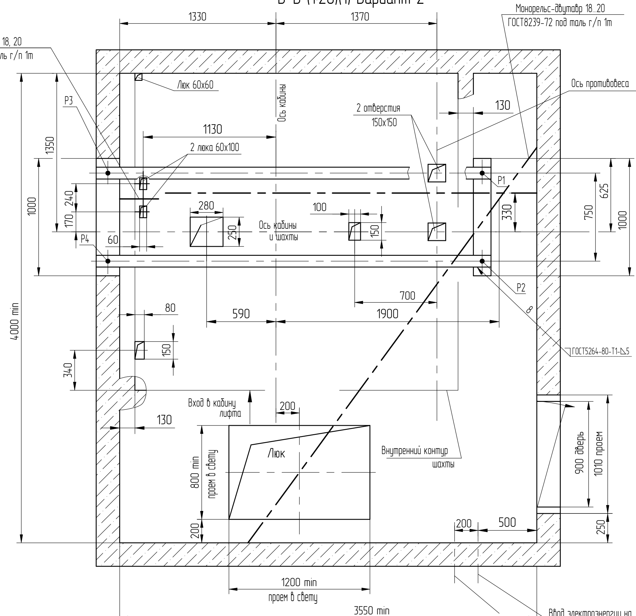
В-В (1:20)(1) Вариант 2
