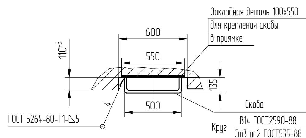
Ю-Ю (1:20)
