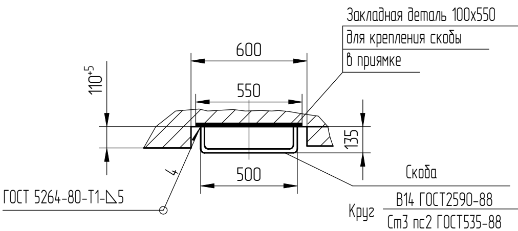
Ю-Ю (1:20)
