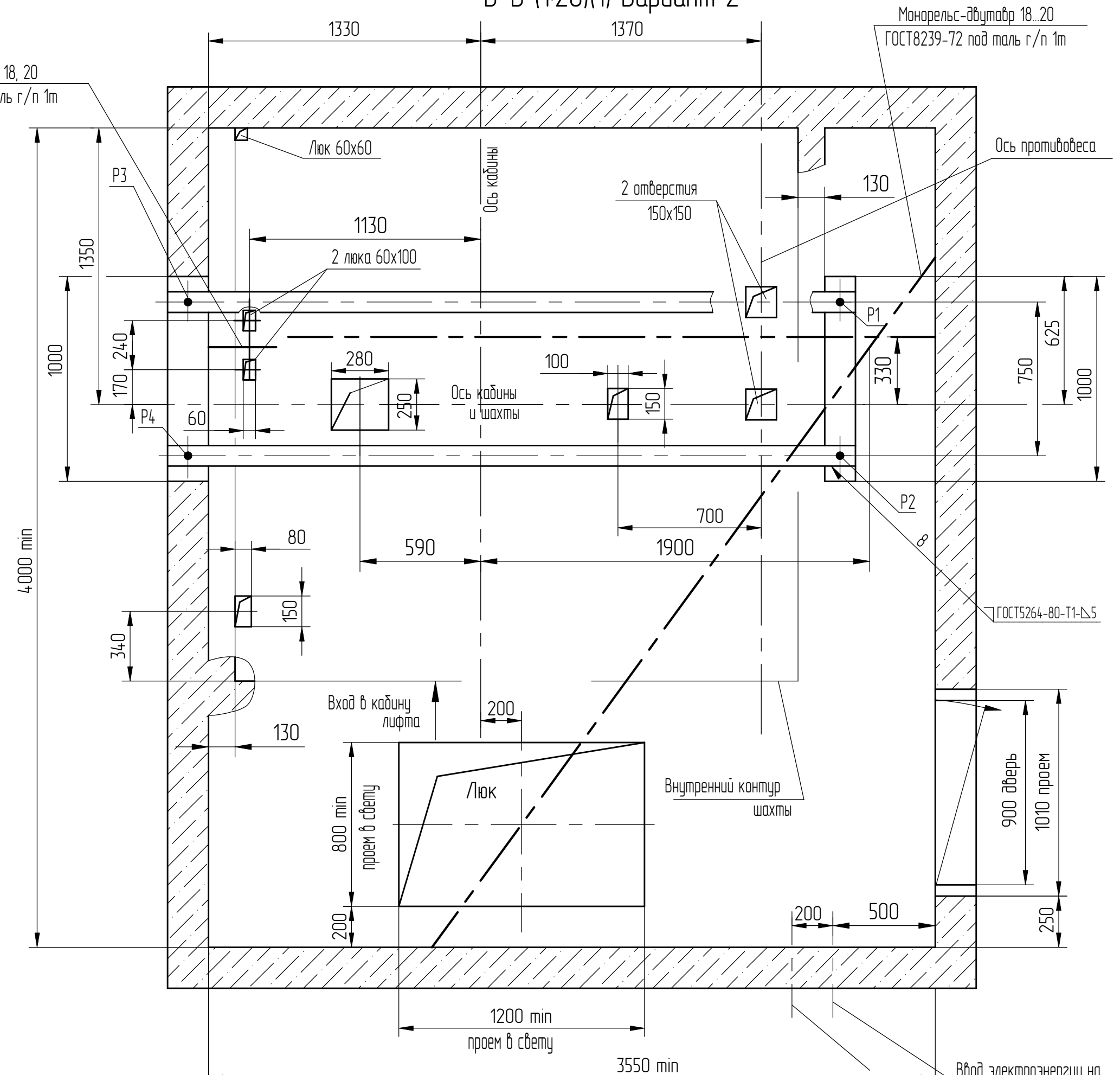
В-В (1:20)(1) Вариант 2
