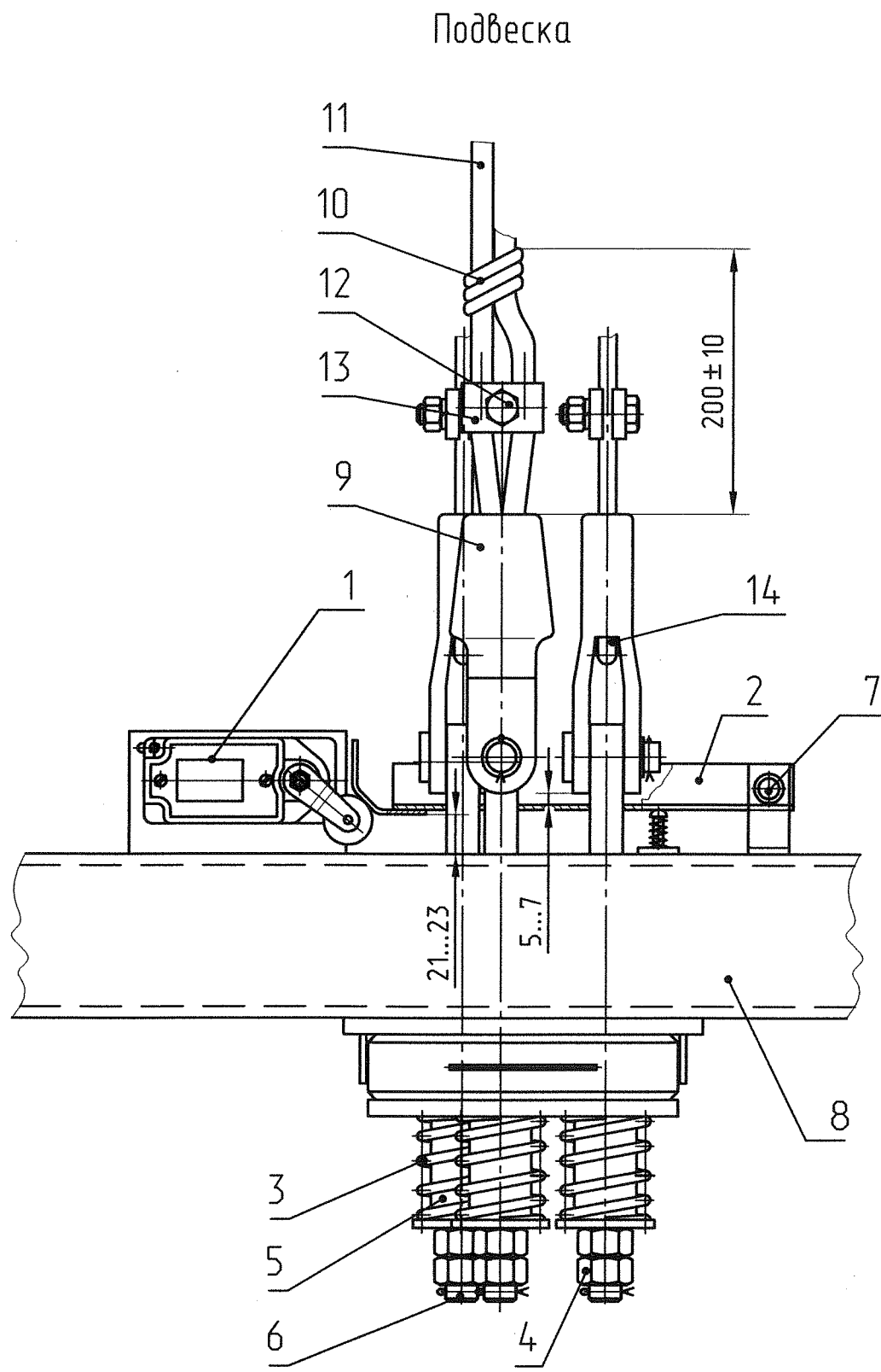
1- Выключатель; 2- лыжа; 3- пружина; 4- гайка; 5- стакан; 6- тяга; 7- ось; 8- балка верхняя; 9- обойма клиновая; 10- проволока; 11- канат; 12- болт; 13- пластина; 14- клин.
