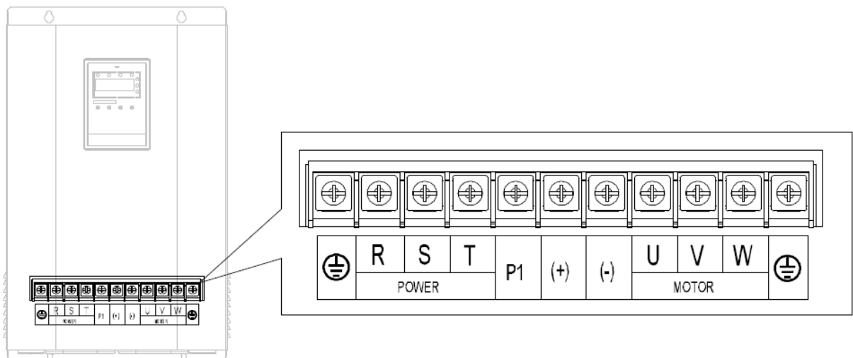
Рисунок 5.3 Общий вид силовых клемм (18кВт-30кВт)
