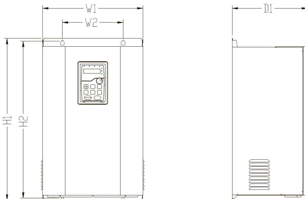
Рисунок 3.3 Конструкция 2
