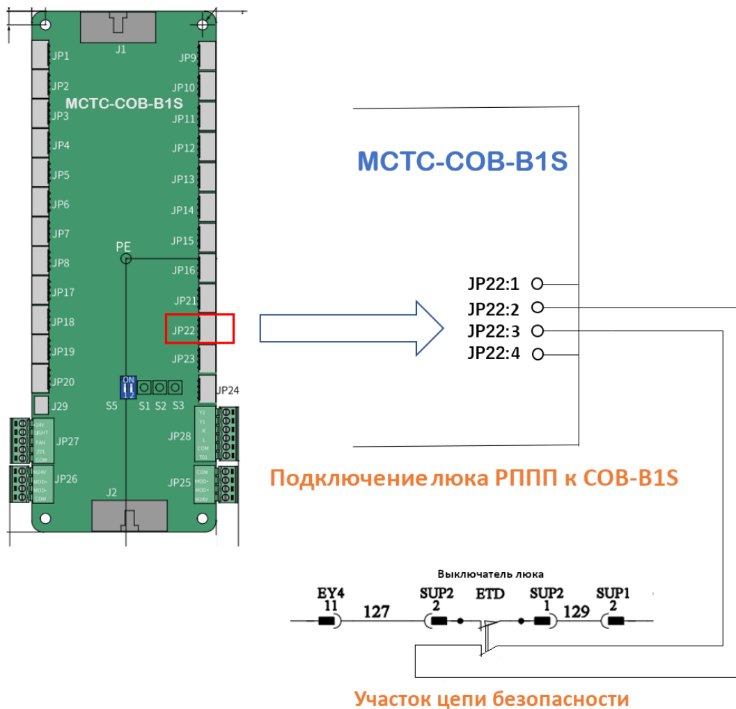
Рисунок 2.6 Подключение выключателя люка в цепь безопасности
