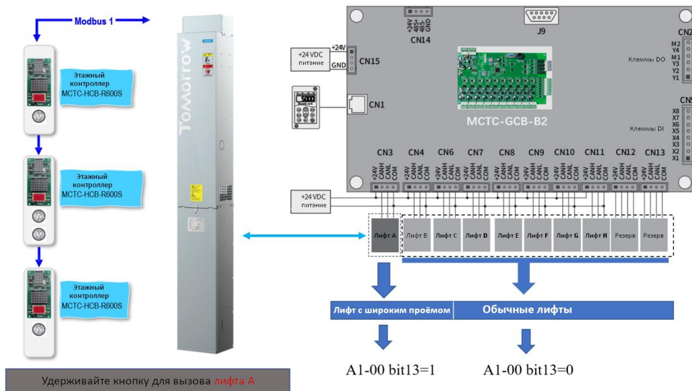
Рисунок 2.3 Схема группового управления
