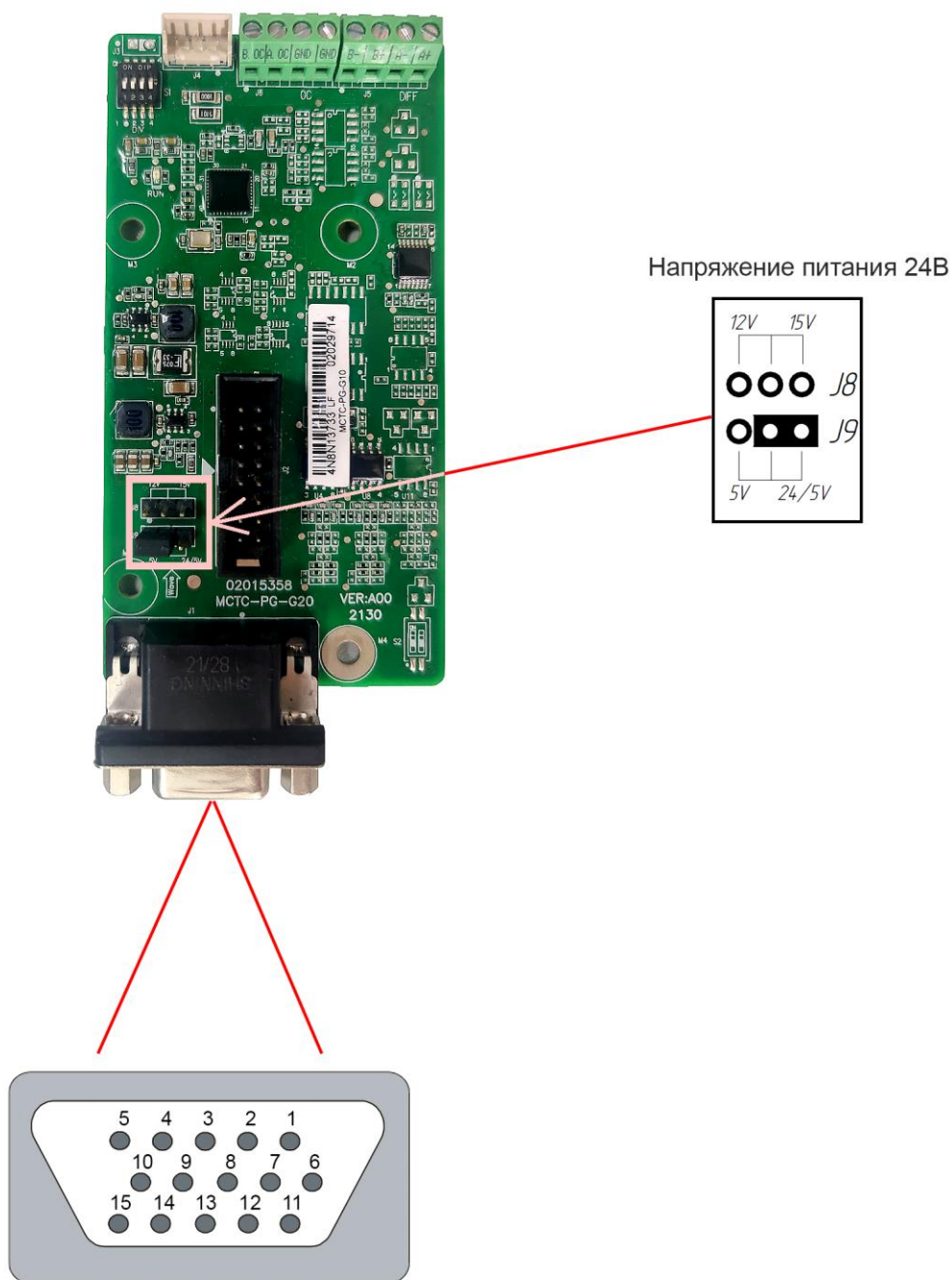
Рисунок 5.4 – Плата подключения энкодера MCTC-PG-G10
