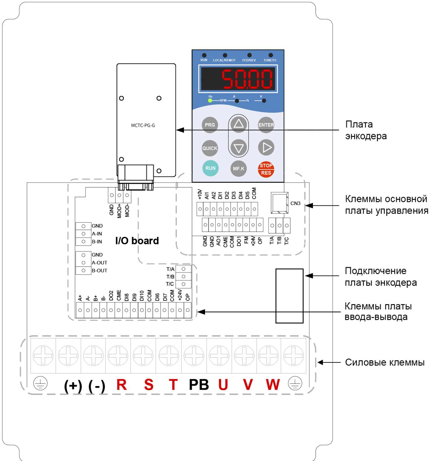
Рисунок 5.1 Общий вид клемм преобразователя частоты
