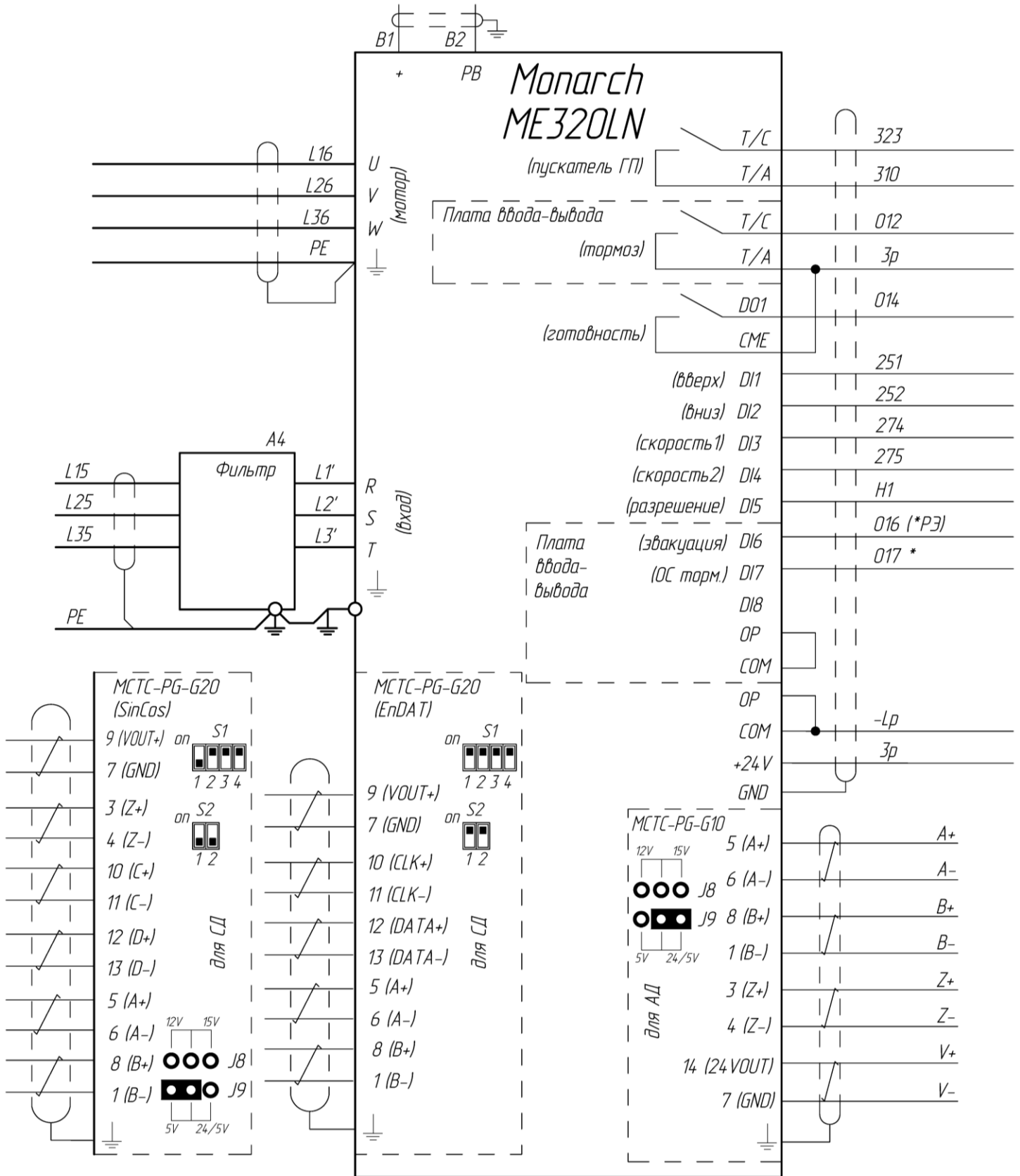
Рисунок 5.2 – Схема подключения к станции УЛ
